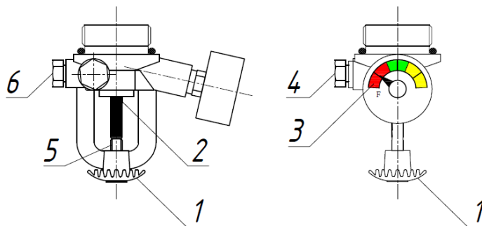
Рисунок 2. Запорно-пусковое устройство
