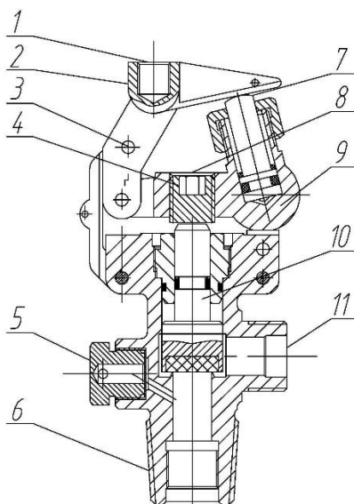
Рисунок 2. Конструкция запорно-пускового устройства для модулей CO 2 :
