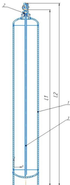
Рисунок 1. Модуль газового пожаротушения - Общий вид
